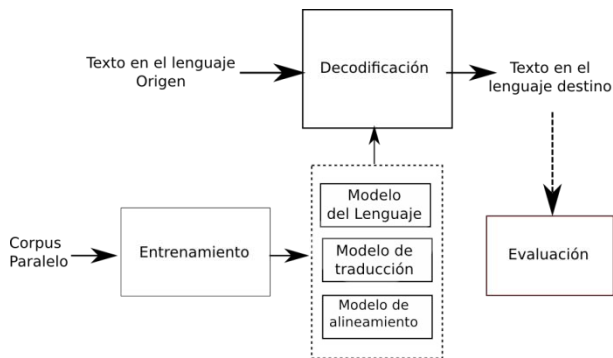
Figura 1: Modelo de un traductor SMT
