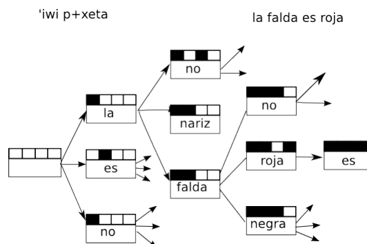
Figura 5: Búsqueda en el espacio de traducción
