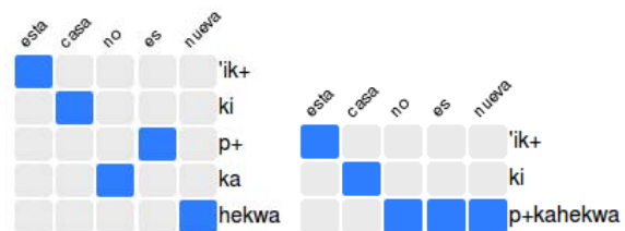
Figura 2: Búsqueda de la mejor traducción
