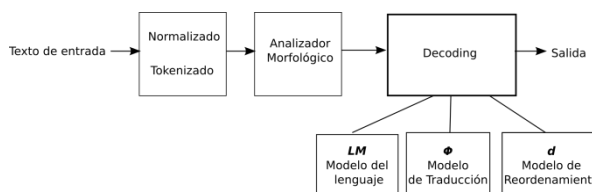
Figura 4: Flujo de traducción
